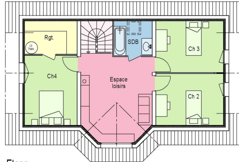
Etage
